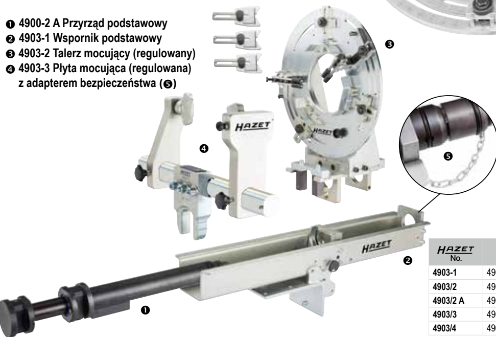
Ściągacz do sprężyn 4903/4
